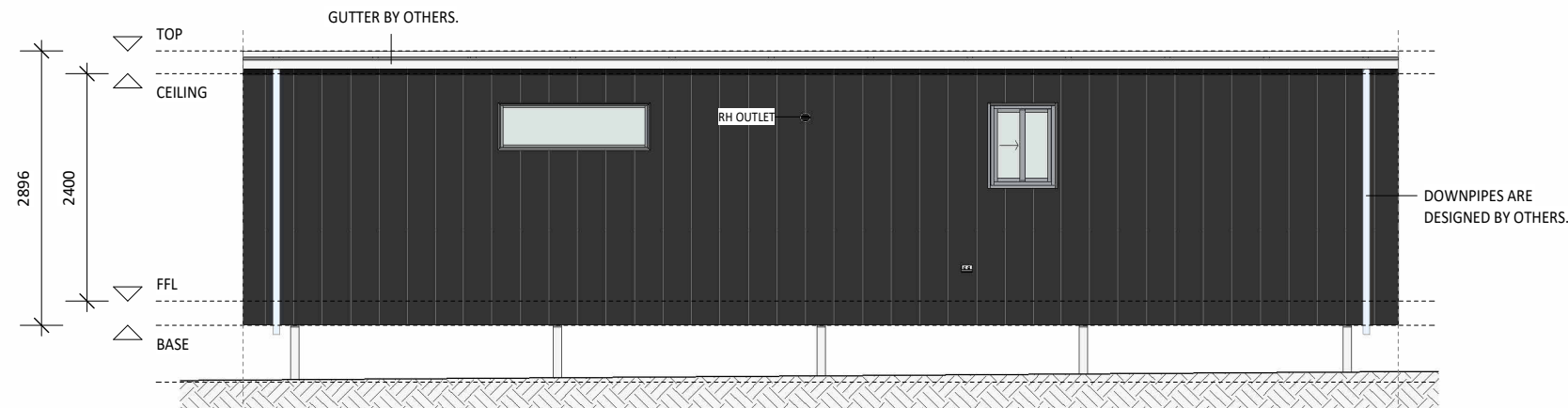
E3 100 scale 1:75 ELEVATION 3
